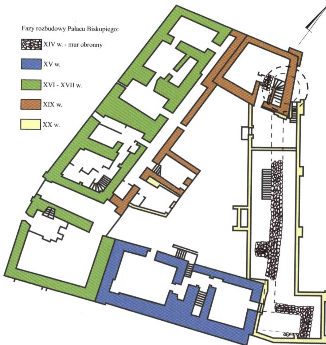
Rys 1. Rzut piwnic kompleksu budynków Pałacu Biskupiego wraz ze średniowiecznym murem obronnym i basztami z oznaczeniem faz rozbudowy. Opr. Z. Gil. M. Pawłowska ( źródło: Pałac Biskupi w Krośnie, dzieje i ewolucja budowli na przestrzeni wieków. Z. Gil )
