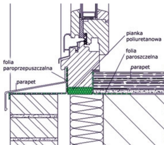
Rys. Montaż parapetu zewnętrznego
